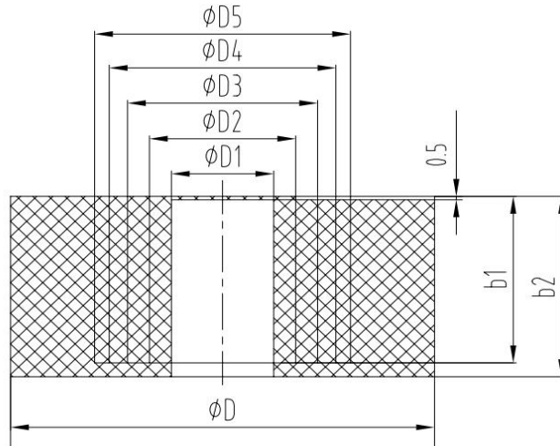
密封圈尺寸 表 5
